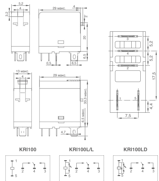
KRI100 Размеры (мм)
