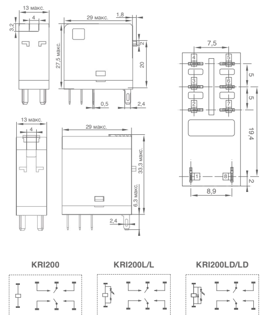
KRI200 Размеры (мм)
